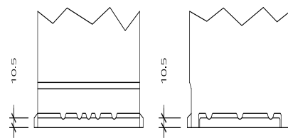
Bodenleiste B13
